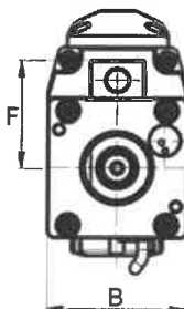
DIN 5482 abgewinkelt 90°, zurückgesetzt DIN 5482 angular 90°, offset
