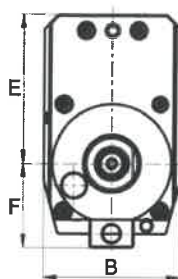
DIN 5482 gerade, versetzt DIN 5482 straight, offset
